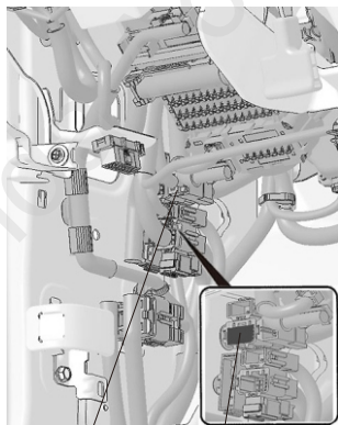
车辆25极连接器
